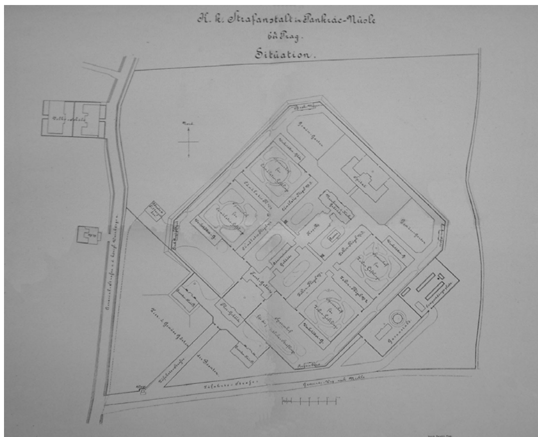
Situační plán c.k. mužské trestnice v Praze (Pankrác – Nusle) z roku 1890
