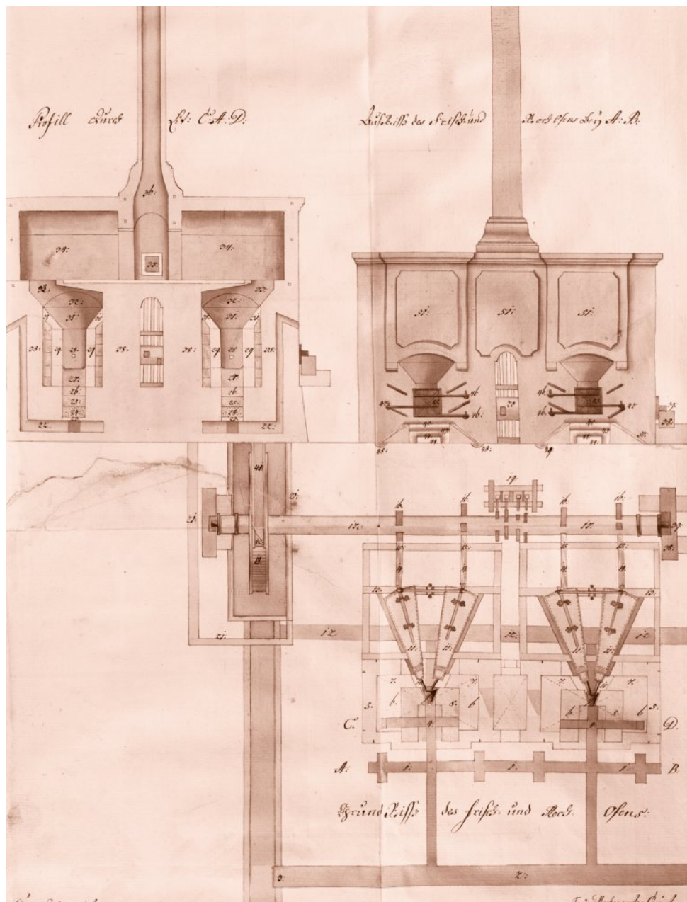
KREMICKÁ SČERSTVOVACIA PEC A PEC NA SUROVÉ SPRACOVANIE RUDY
