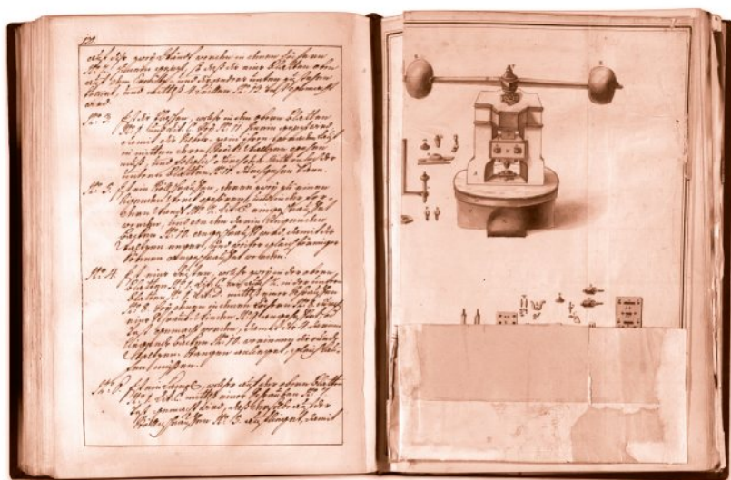
MINCIARSKÉ TECHNICKÉ ZARIADENIA A ICH PODROBNÝ POPIS NA STRÁNKACH ZLATEJ KNIHY BANÍCKEJ
