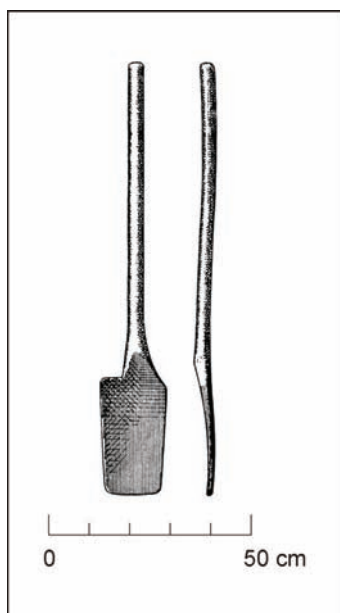
Obr. 4. Celodrevený asymetrický rýľ z Osebergu, Nórsko, 9.-10. storočie. (cit. podľa Szabó/Grenander-Nyberg/Myrdal 1985 , obr. 20).
