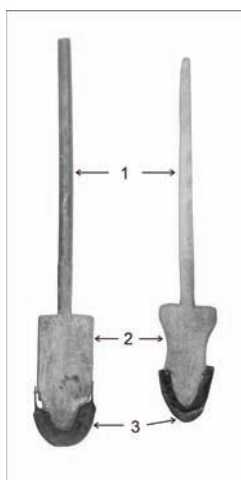
Obr. 1. Drevené rýle so železným okutím z 19. storočia z oblasti Târgu Mureș, Rumunsko. 1 - rukoväť, 2 - čepel, 3 - železné okutie.
